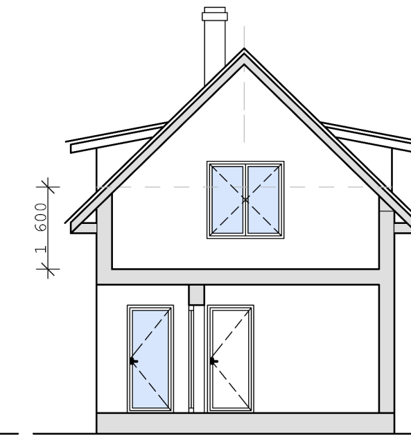
Lõige 1. M 1 : 100
