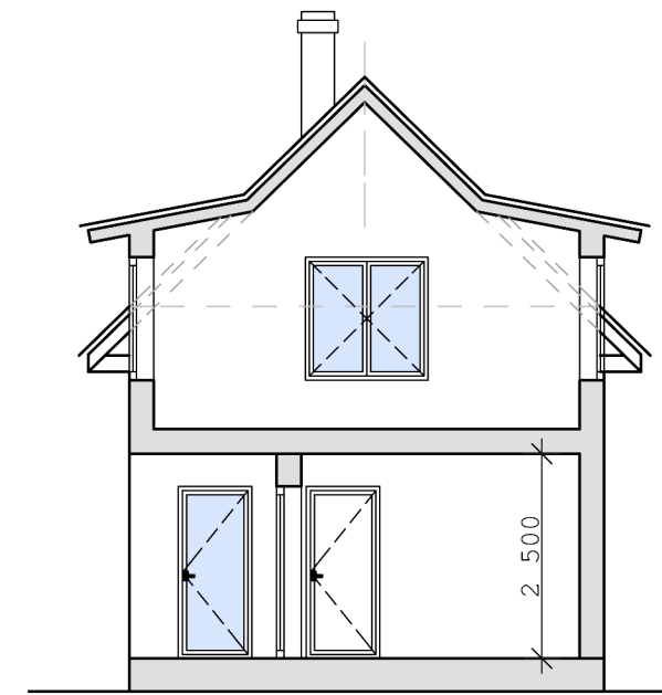
Lõige 2. M 1 : 100
