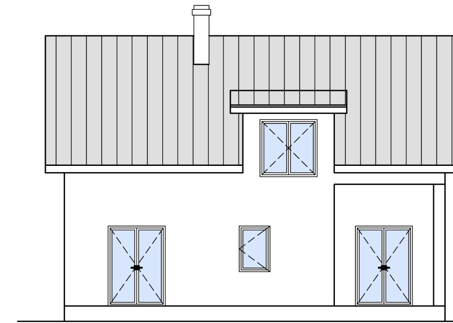
Fassaad A. M 1 : 100
