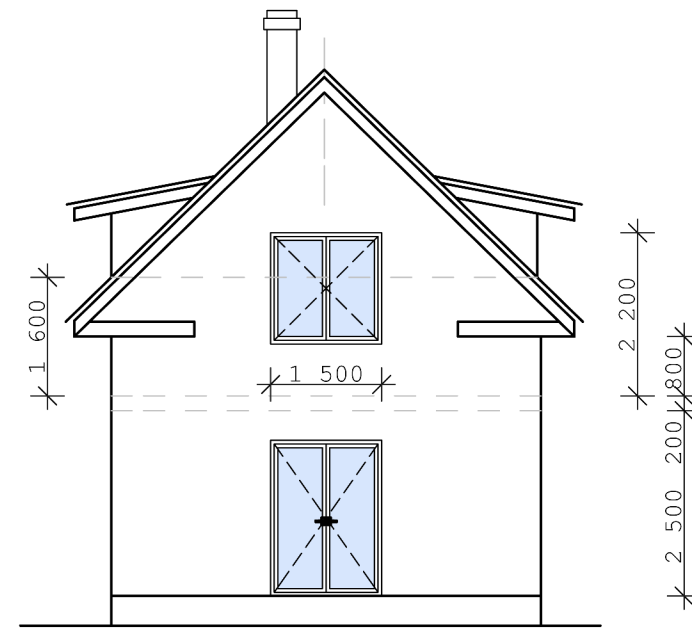
Fassaad B. M 1 : 100
