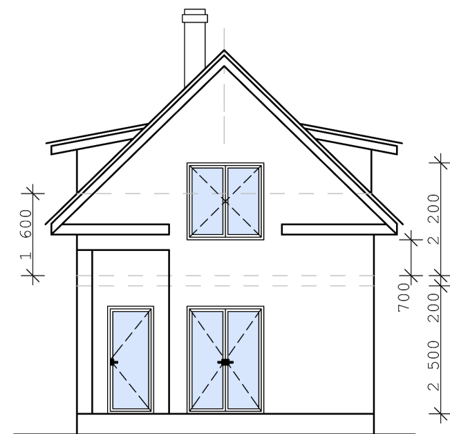
Fassaad D. M 1 : 100
