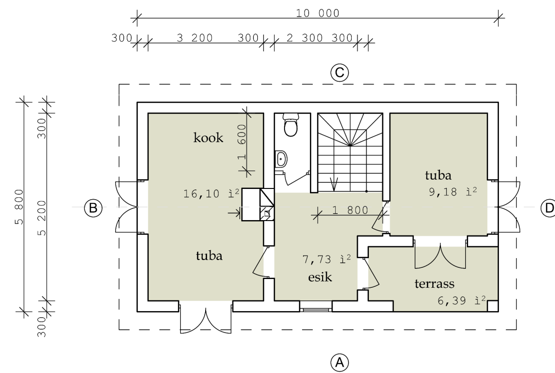
Aiamaja 1. korruse plaan. M 1 : 100
