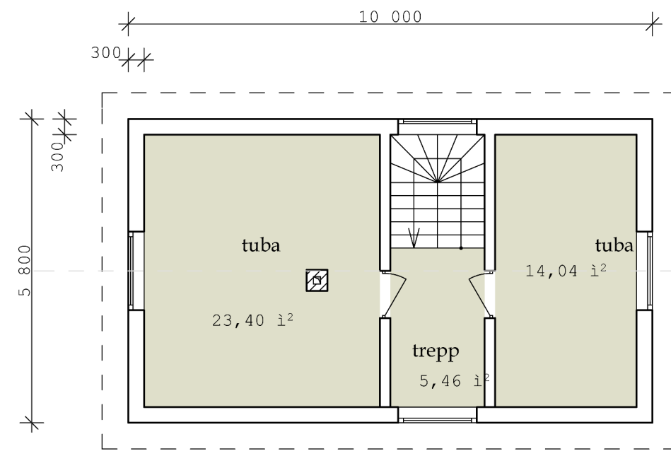
Mansardi korruse plaan. M 1 : 100
